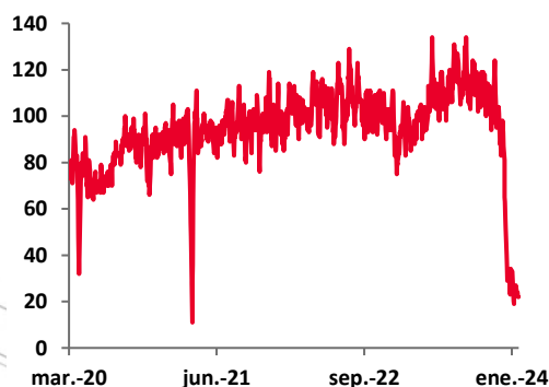
Flujo de buques comerciales en el Canal de Suez Buques por semana
